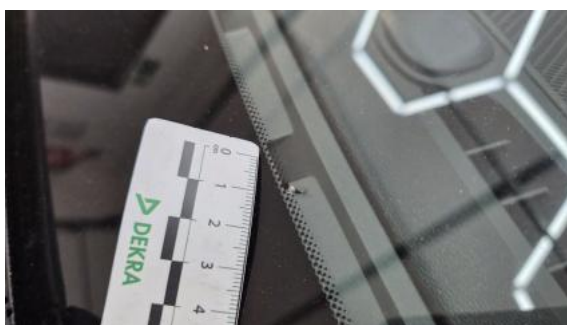
Fot. 39 Szyba czołowa - Pęknięcie/rozerwanie 1
