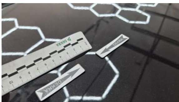
Fot. 35 Pokrywa komory silnika - Wgniecenie/odkształcenie 1
