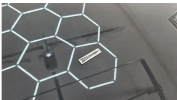
Fot. 37 Pokrywa komory silnika - Wgniecenie/odkształcenie 1
